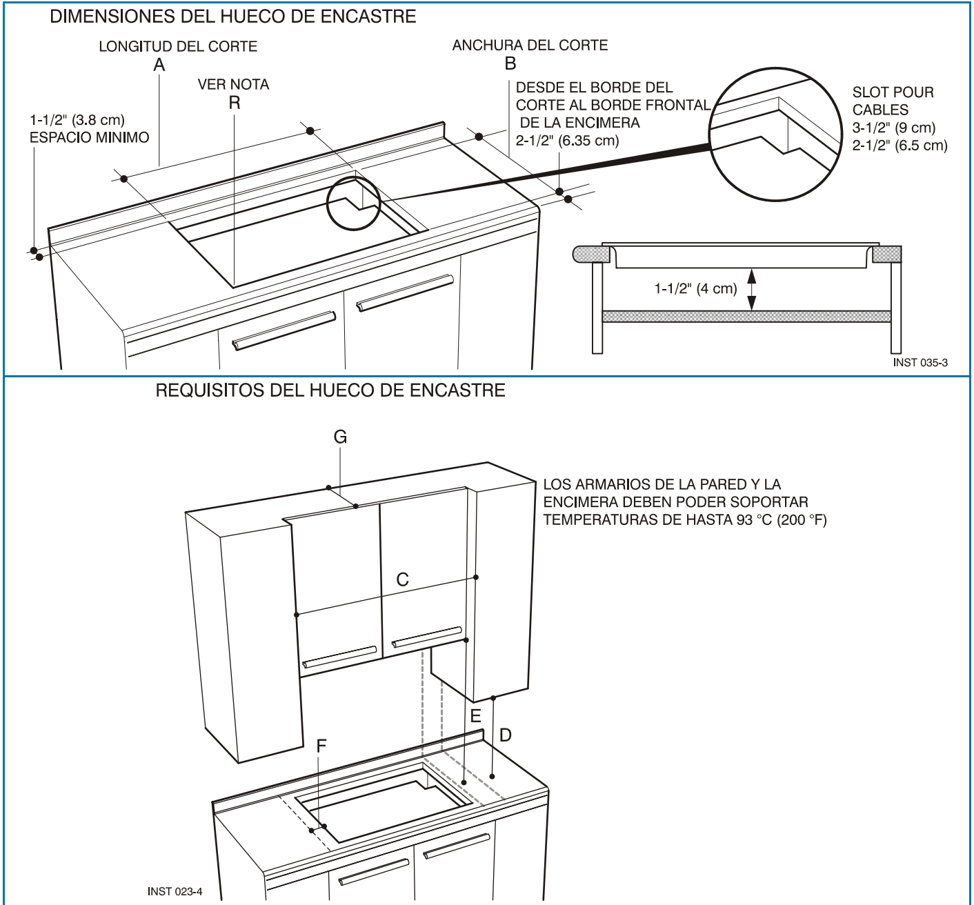
Figura 3. Dimensiones de encastre
